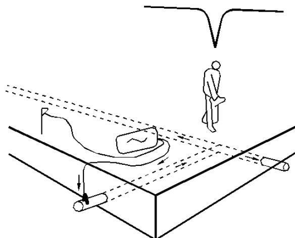
管线追踪示意图
