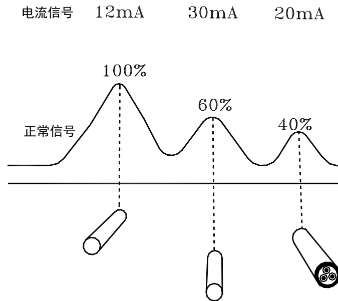
图 f 电流测量示意图
