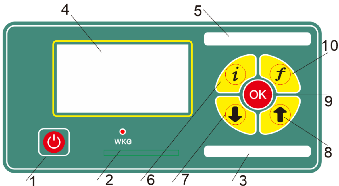
发射机面板示意图
